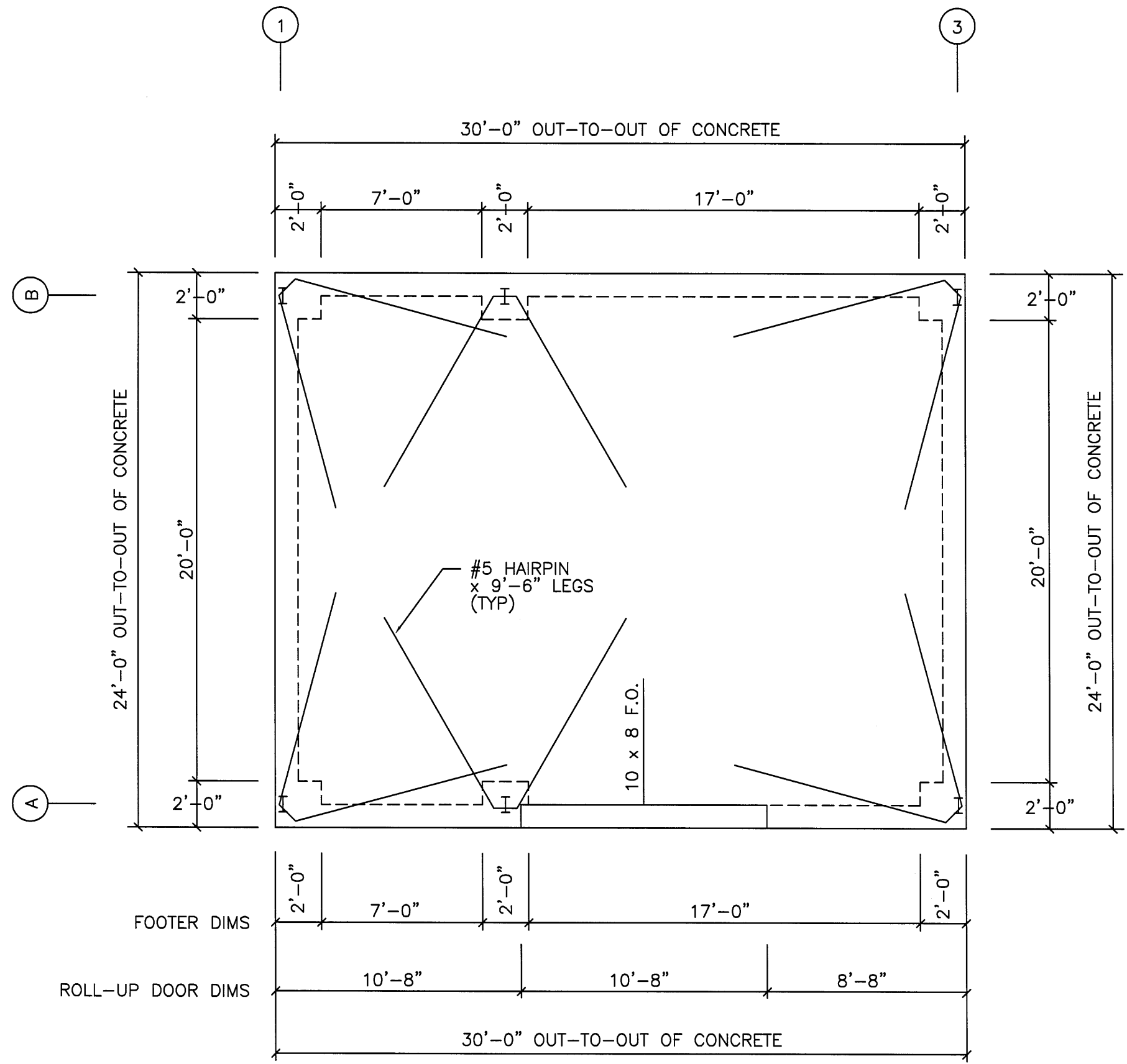
FOUNDATION PLAN N.T.S.
