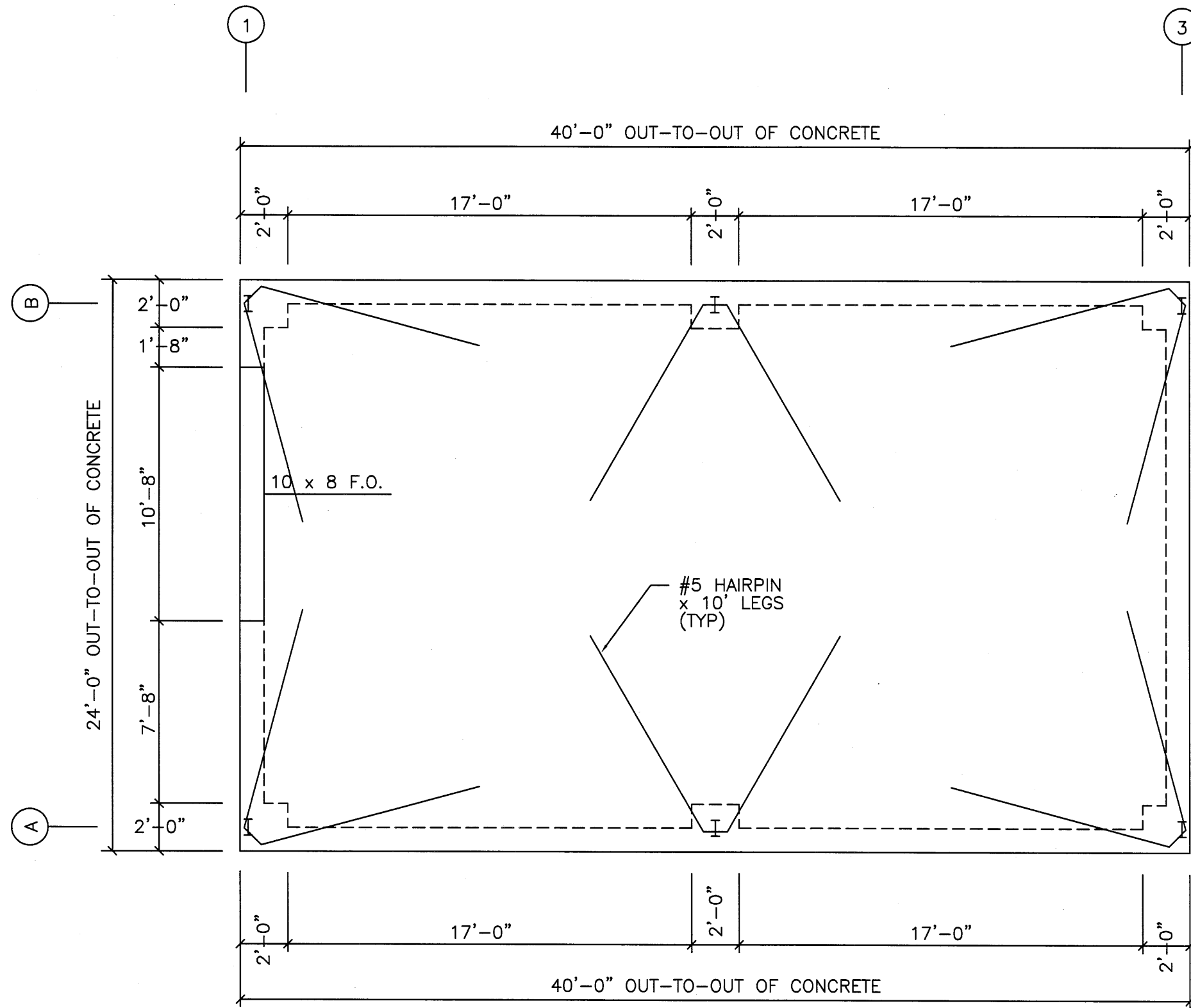
FOUNDATION PLAN N.T.S.
