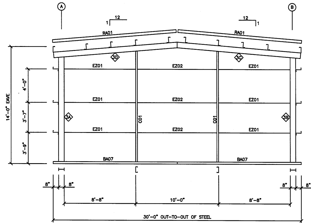
ENDWALL FRAMING ELEV. ● COL. LINE 3 N.T.S.
