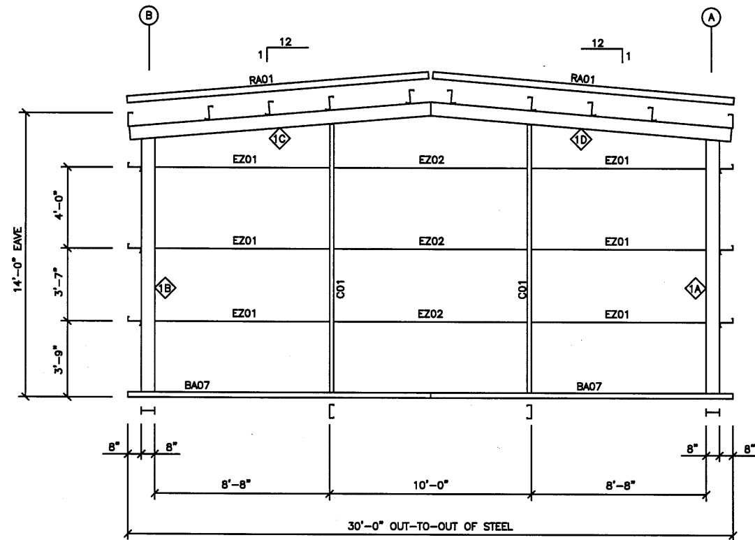
ENDWALL FRAMING ELEV. ● COL. LINE 1 N.T.S.
