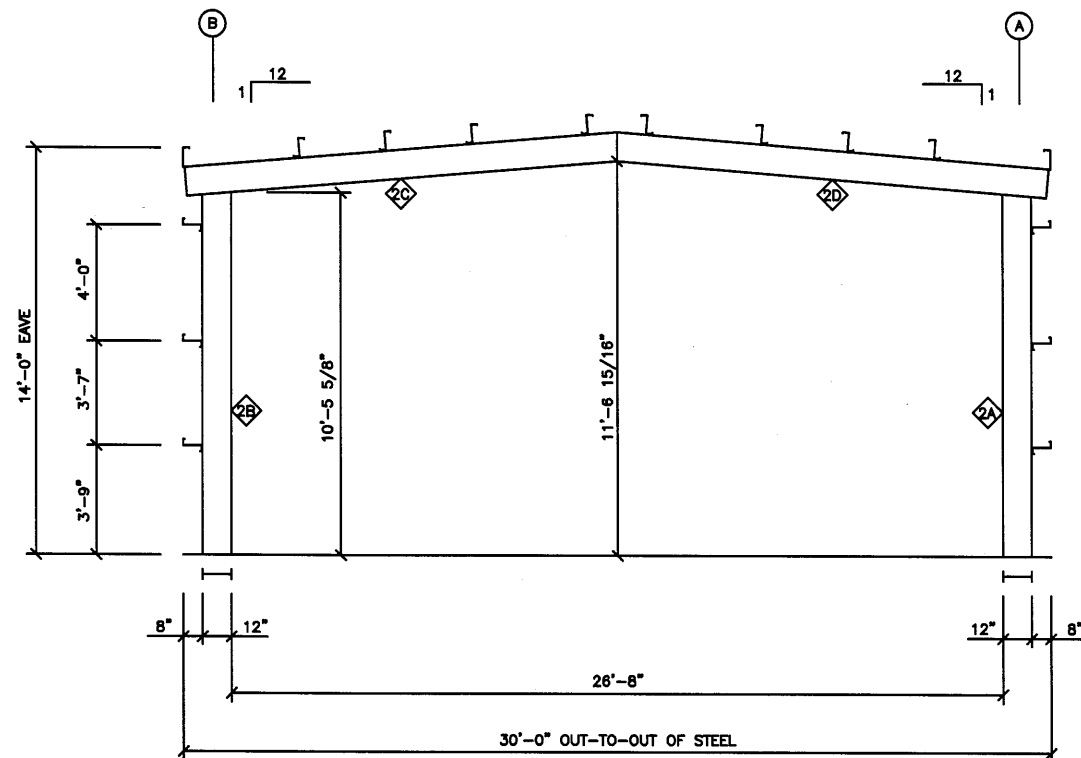
RIGID FRAMING ELEV. ● COL. LINE 2 N.T.S.
