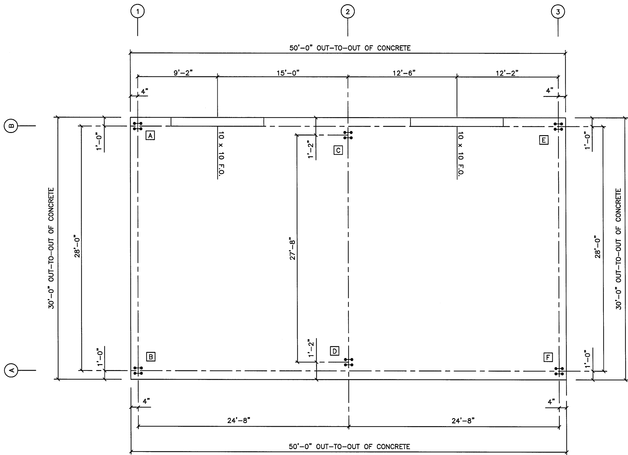
ANCHOR BOLT PLAN N.T.S.
