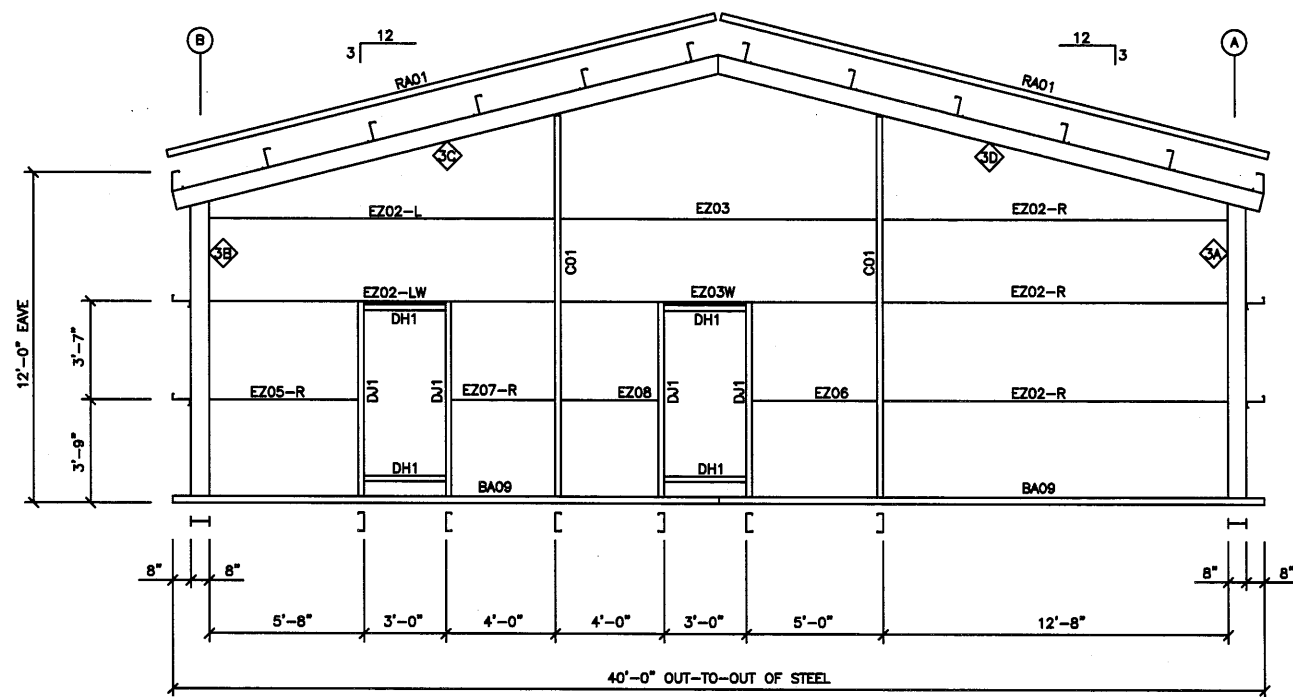
ENDWALL FRAMING ELEV. @ COL. LINE 3 N.T.S.
