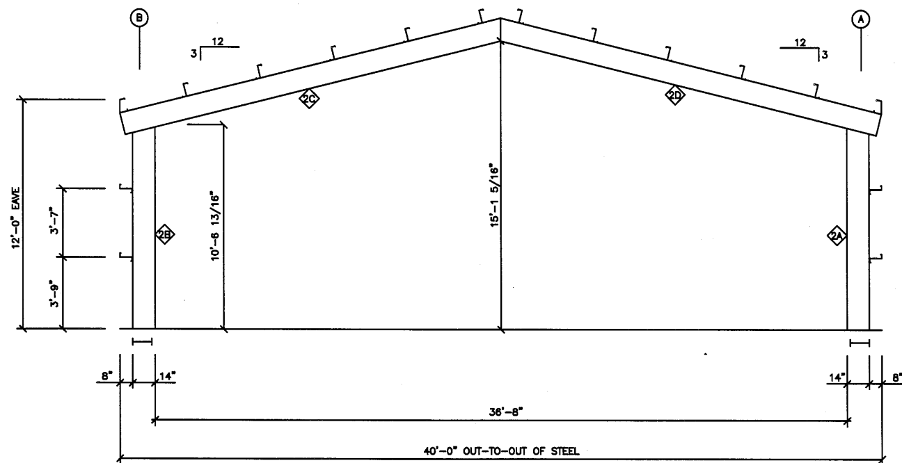
RIGID FRAMING ELEV. @ COL. LINE 2 N.T.S.
