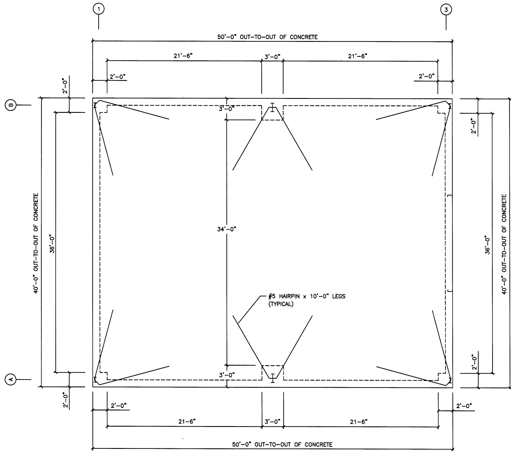
FOUNDATION PLAN N.T.S.
