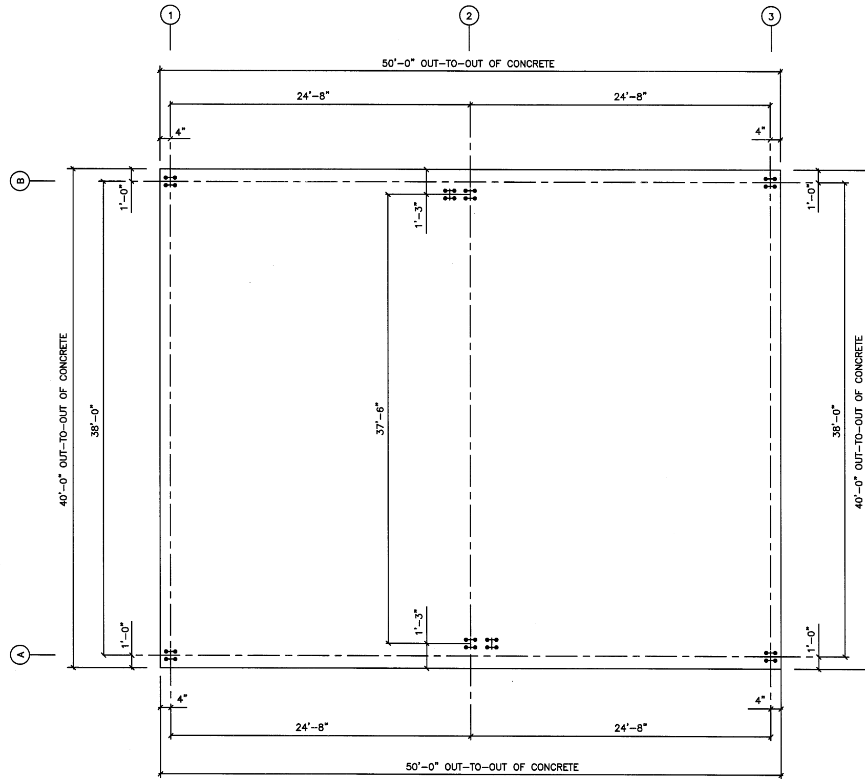
ANCHOR BOLT PLAN N.T.S.
