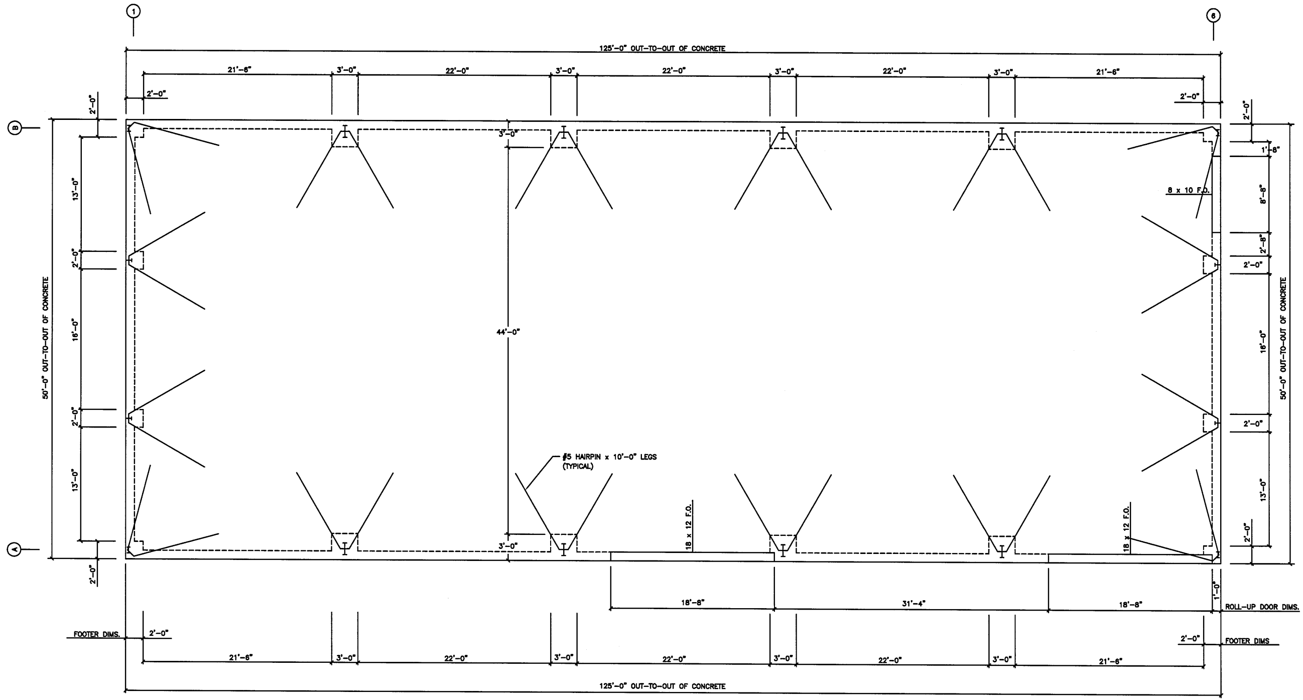
FOUNDATION PLAN N.T.S.
