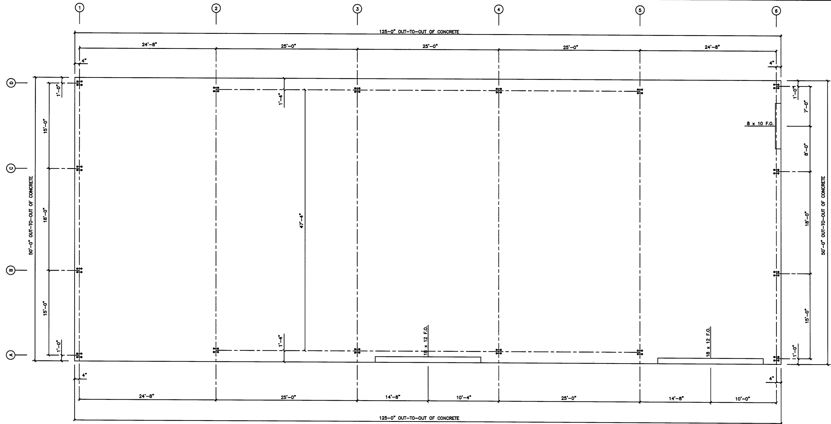
ANCHOR BOLT PLAN N.T.S.
