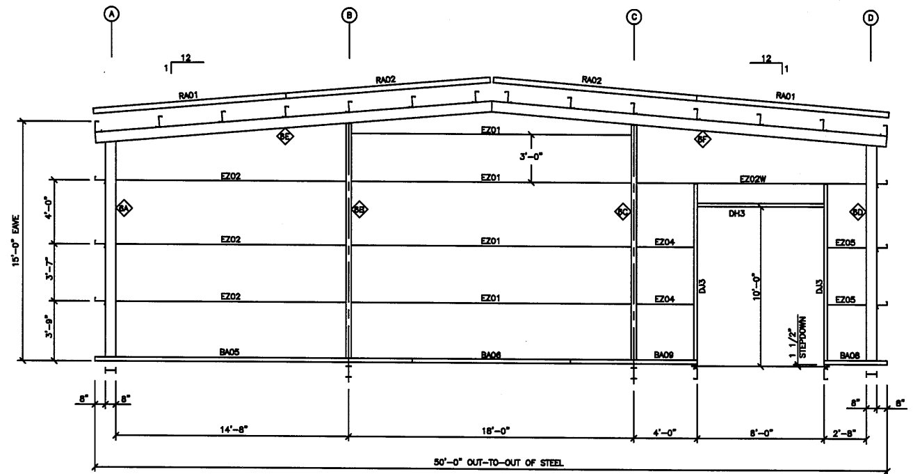
ENDWALL FRAMING ELEV. @ COL. LINE 6 N.T.S.
