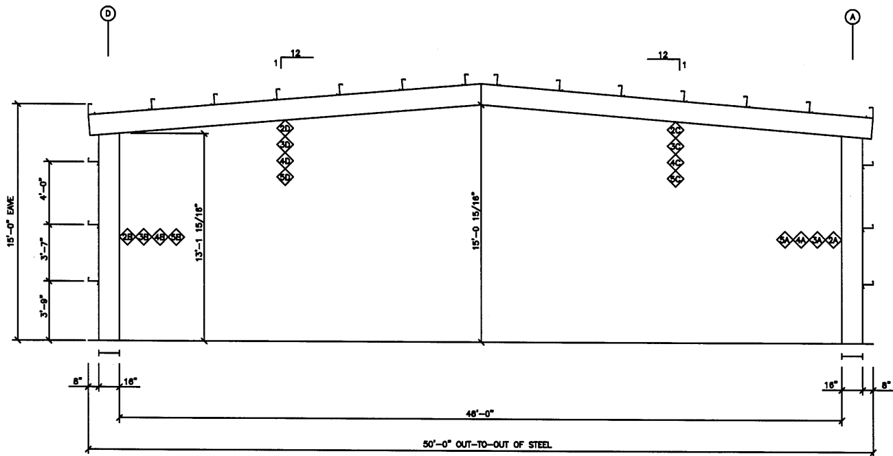
RIGID FRAMING ELEV. @ COL. LINES 3 N.T.S.
