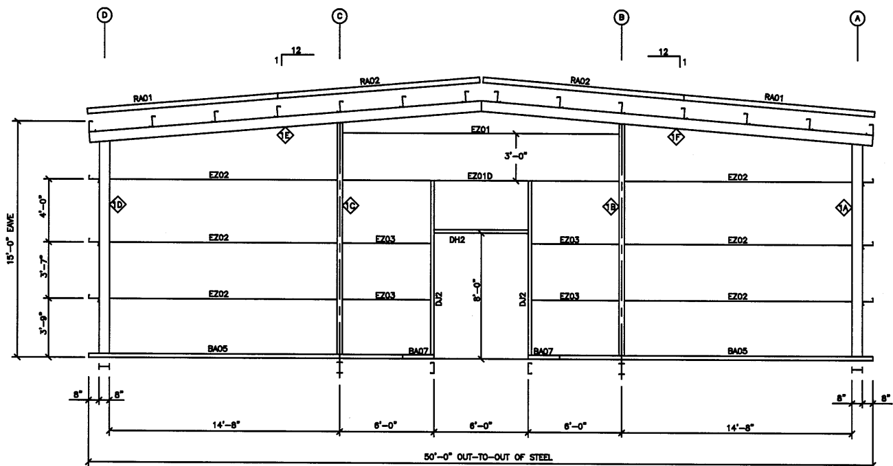
ENDWALL FRAMING ELEV. @ COL. LINE 1 N.T.S.
