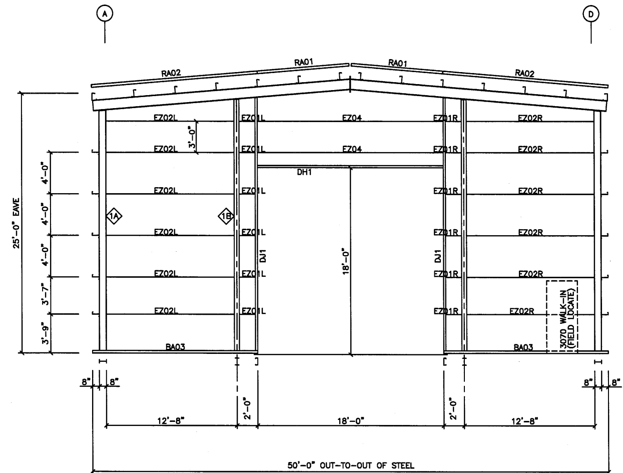
ENDWALL FRAMING ELEV. ● COL. LINE 3 N.T.S.
