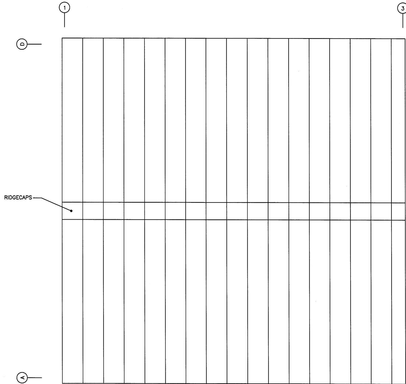
ROOF SHEETING PLAN N.T.S.
