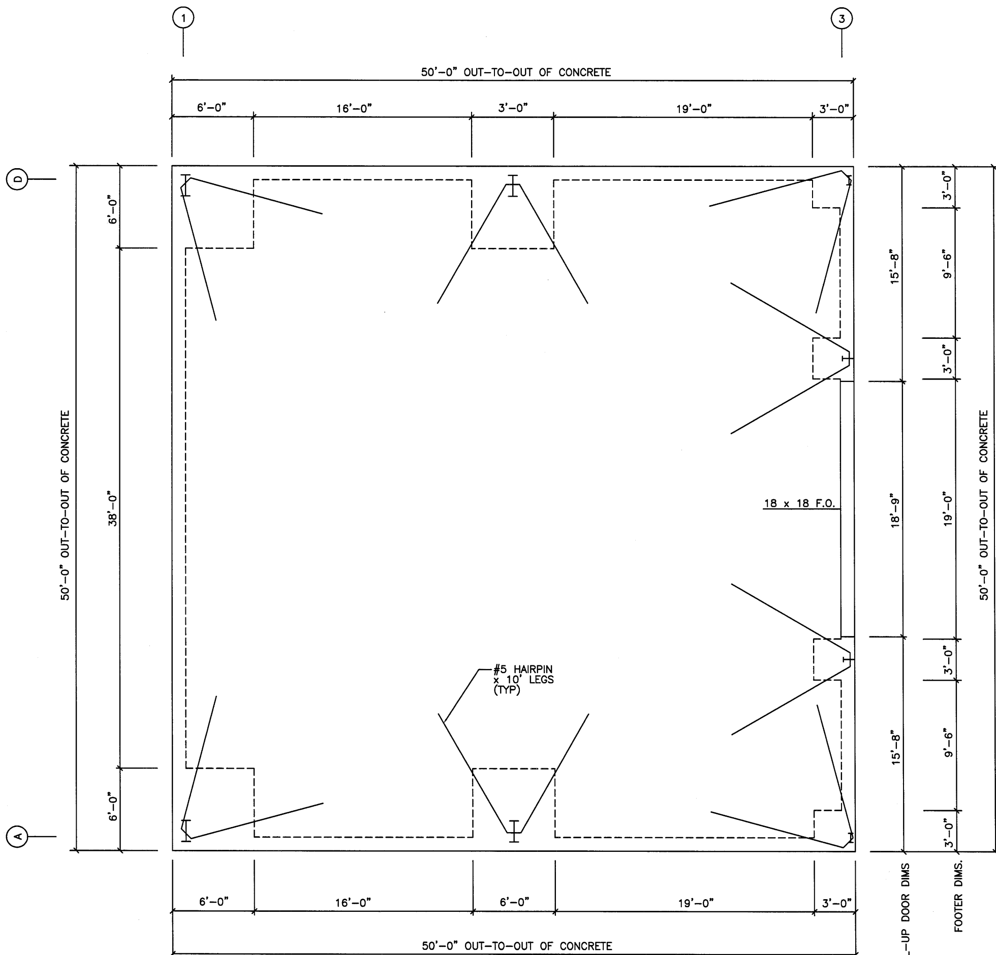
FOUNDATION PLAN N.T.S.
