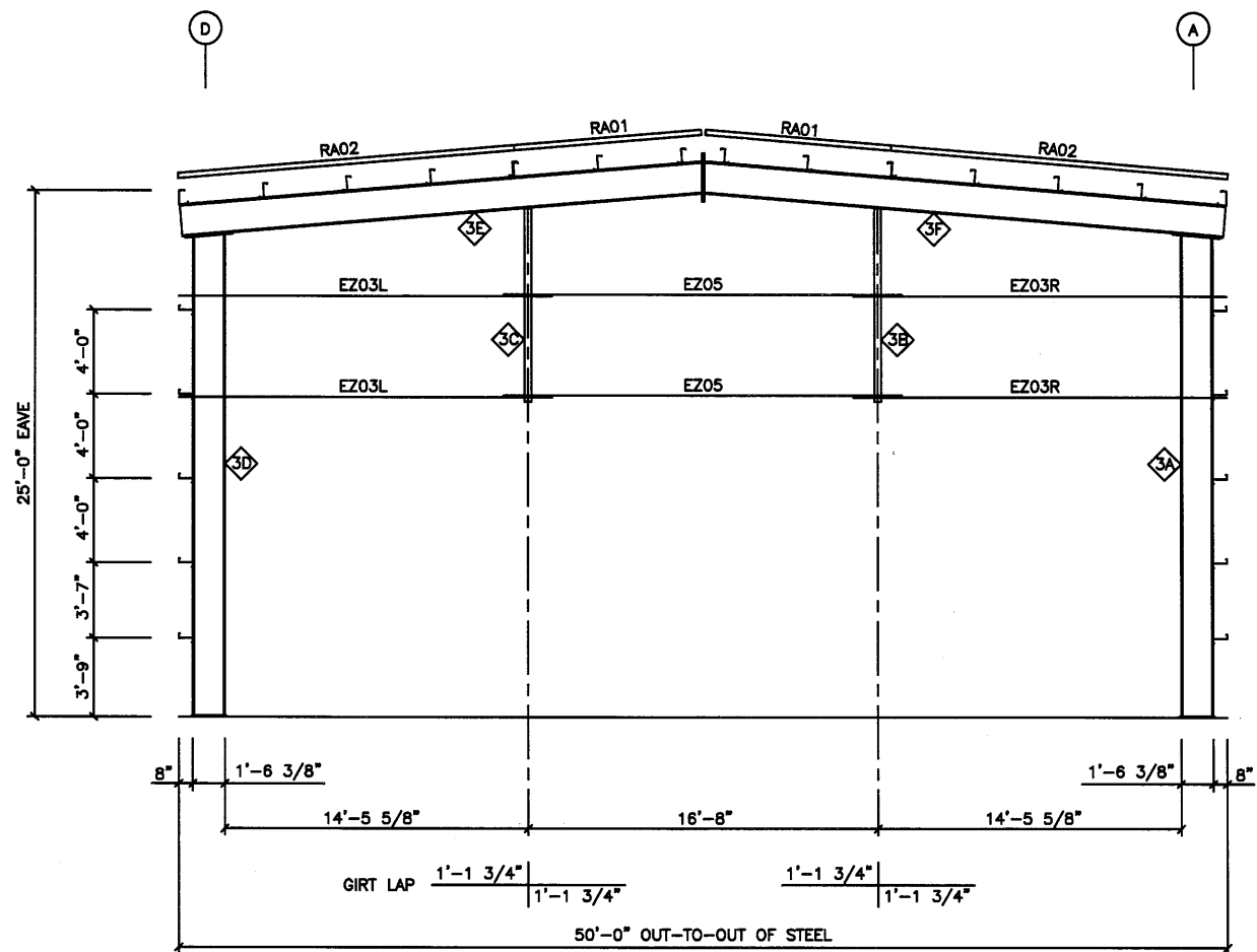
ENDWALL FRAMING ELEV. ● COL. LINE 1 N.T.S.
