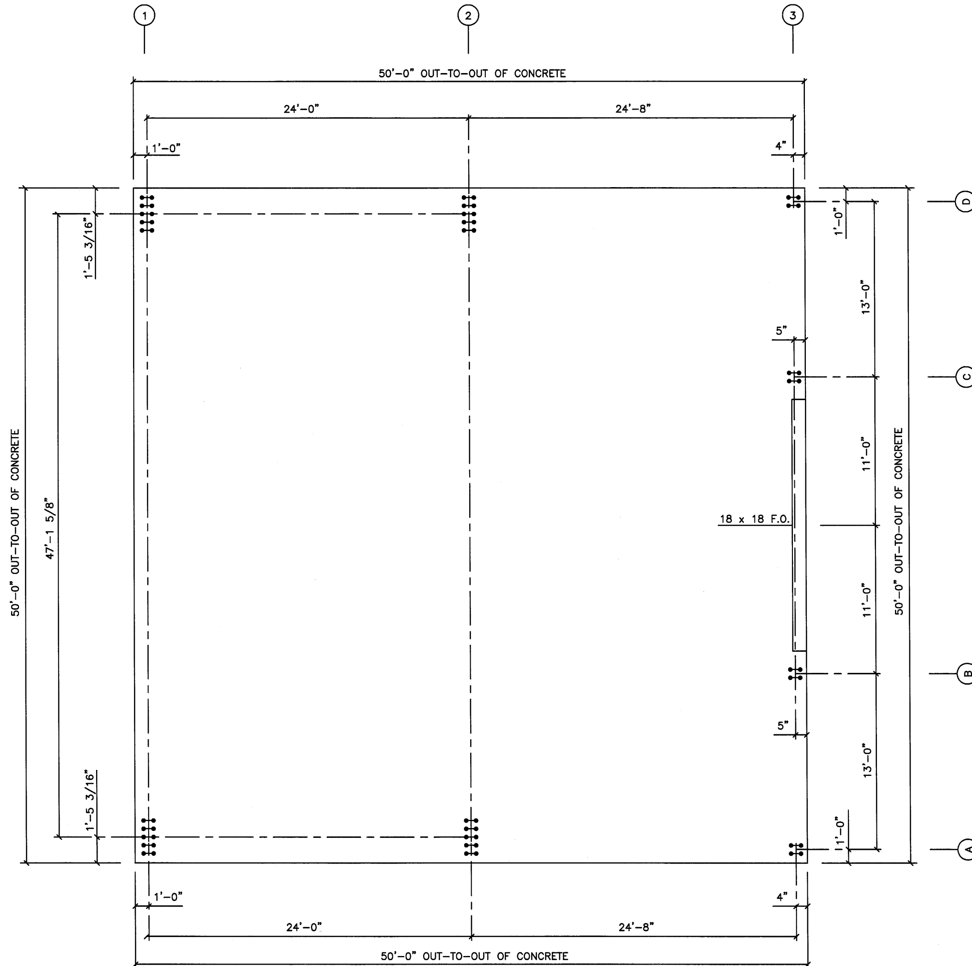
ANCHOR BOLT PLAN N.T.S.
