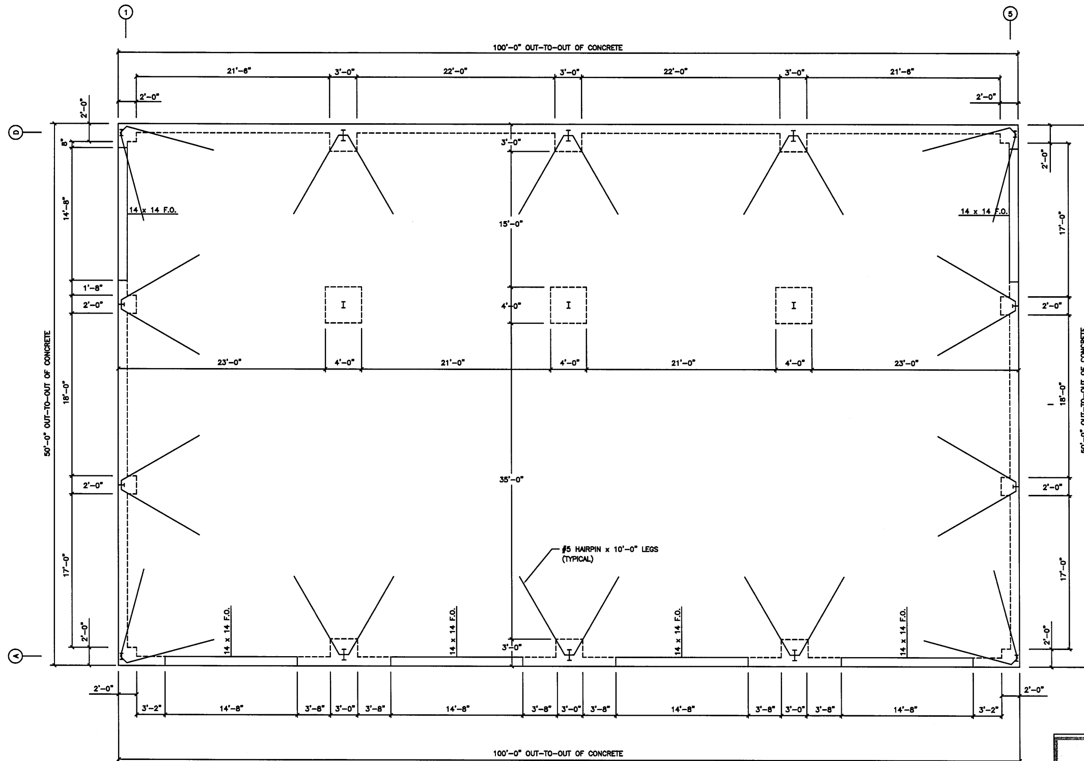
FOUNDATION PLAN N.T.S.
