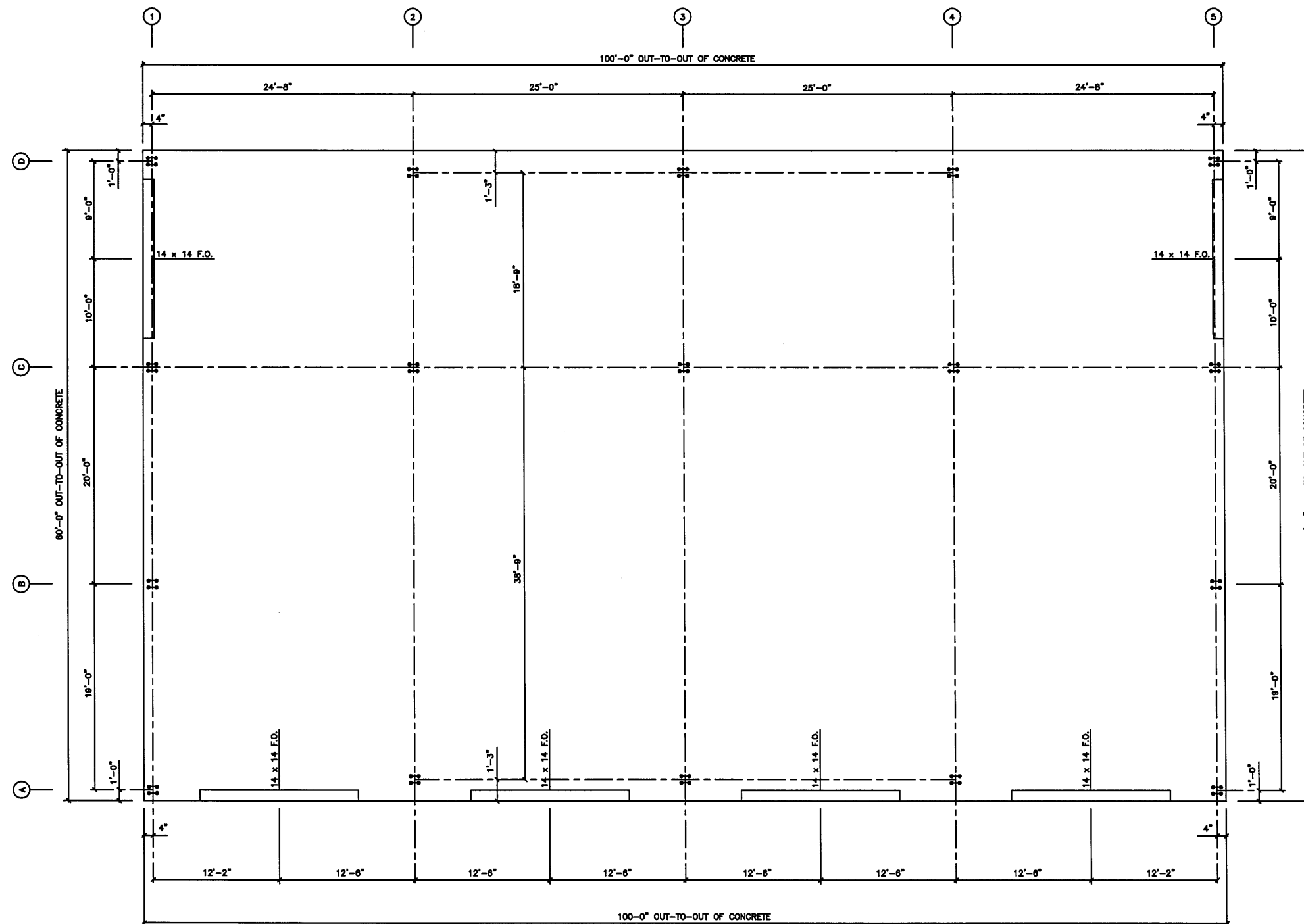
ANCHOR BOLT PLAN N.T.S.
